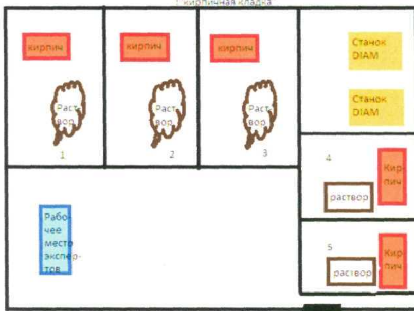
Схема постройки соревновательной площадки по компетенции "кирпичная кладка"
